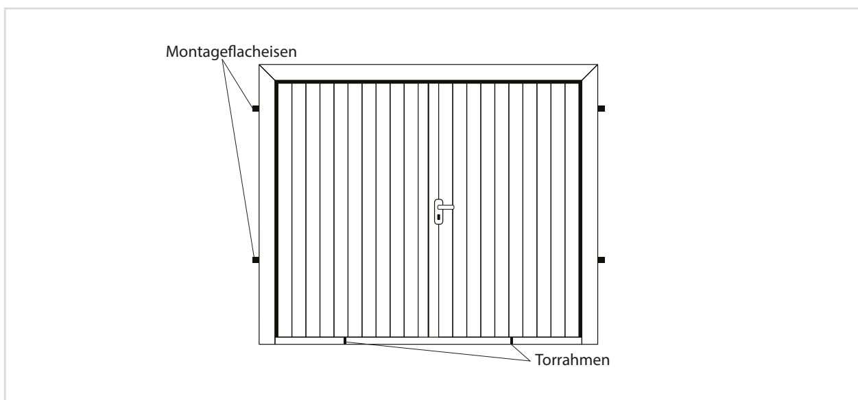
Zeichnung 1 Platzierung der Montageflacheisen
