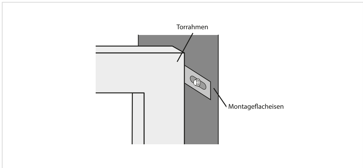
Zeichnung 2 Befestigung des Flacheisens an der Wand
