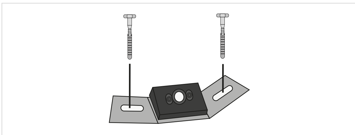
Zeichnung 5 Riegel-Fuß
